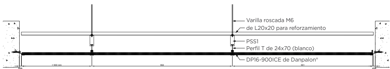
Corte A-A: En área de reforzamiento
